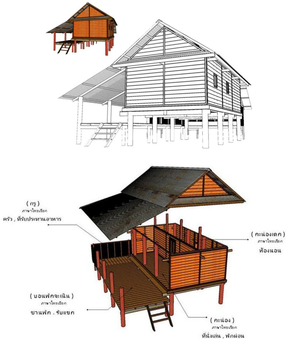
ภาพที่ 5.1 ปะเตียะมาคะนอง (บ้านหนึ่งหลัง)
