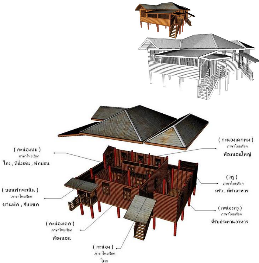
ภาพที่ 5.4 ปะเตียะปัญญา (บ้านปั้นหยา)
