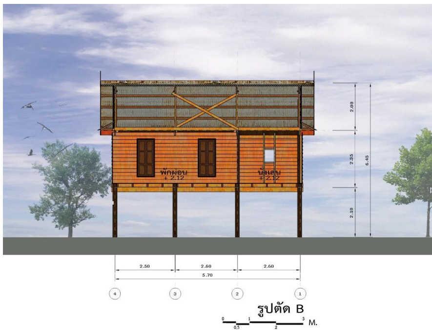
ภาพที่ 5.12 รูปตัด B
