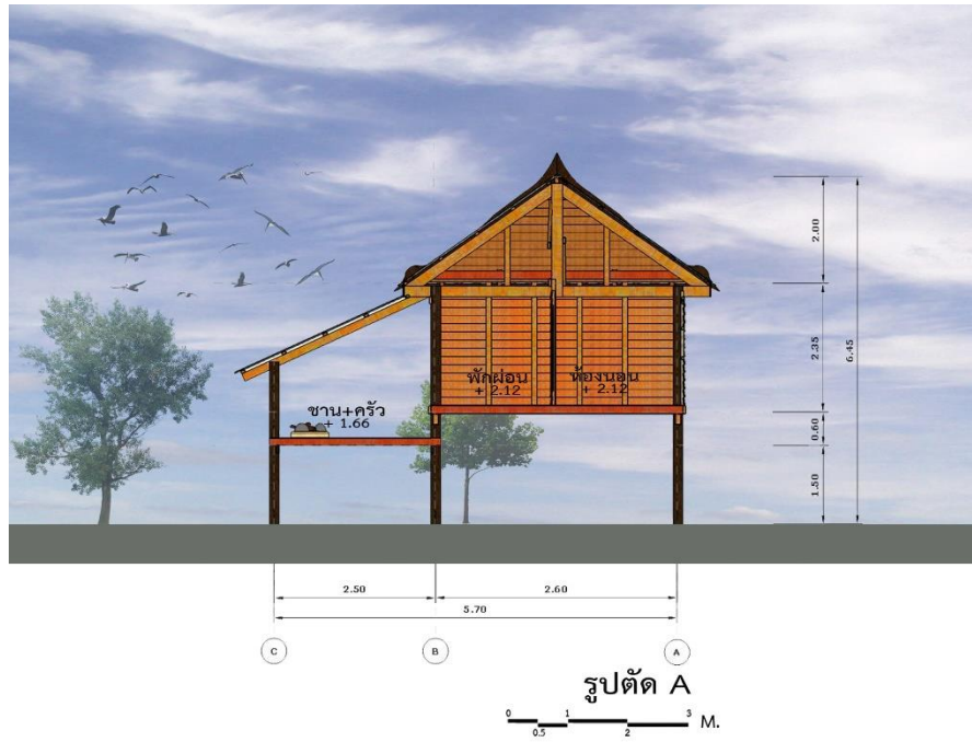
ภาพที่ 5.11 รูปตัด A
