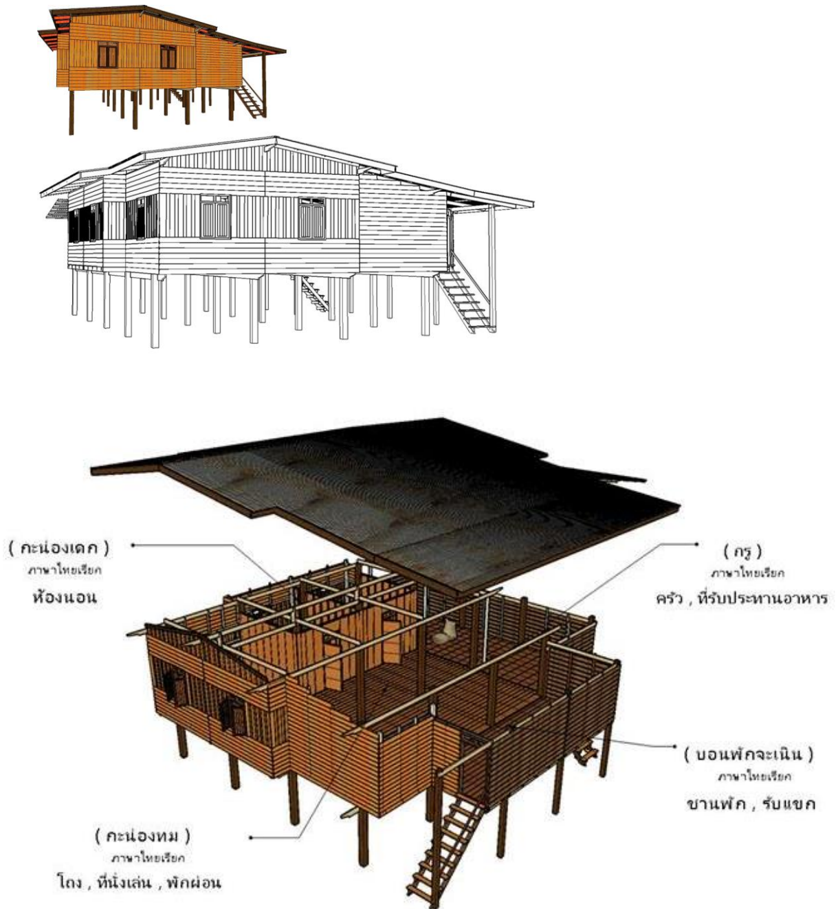
ภาพที่ 5.3 ปะเตียะทม (บ้านหลังใหญ่)
